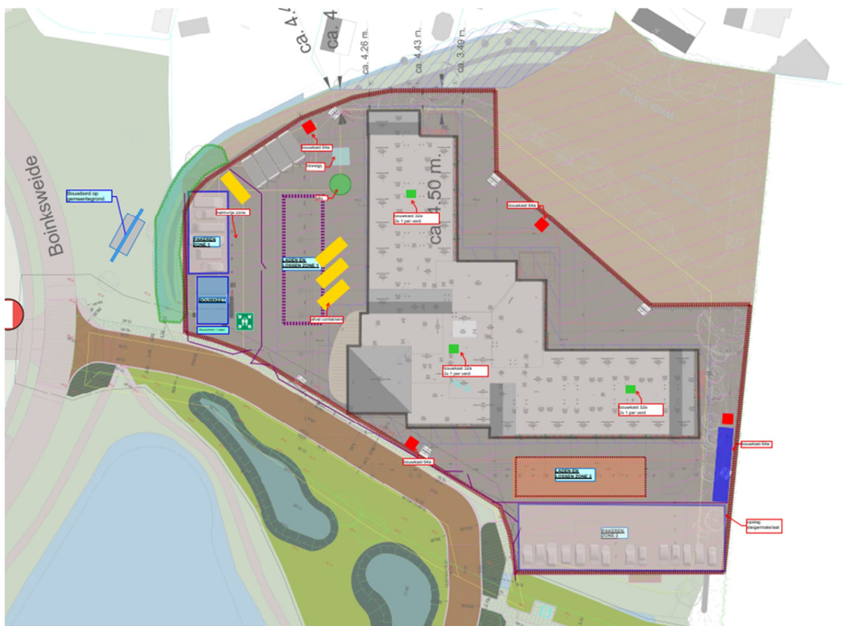
- Bovenaanzicht van de bouwplaats -
